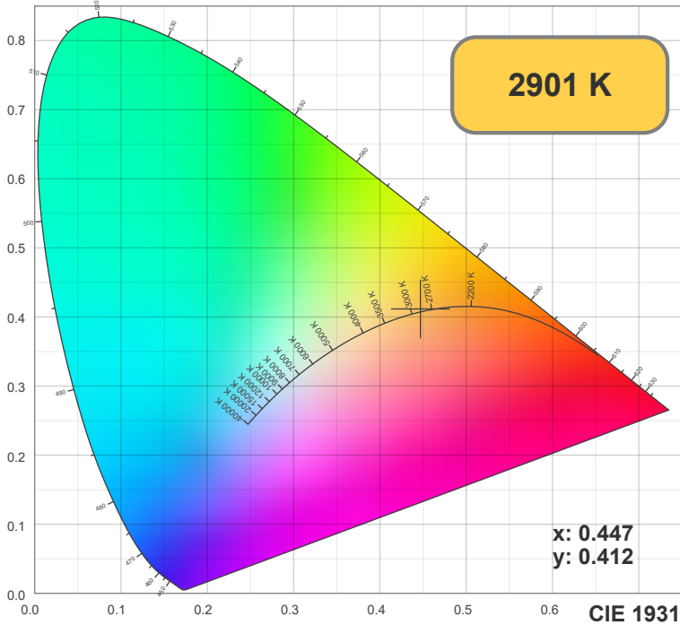
TM30: 91.1
