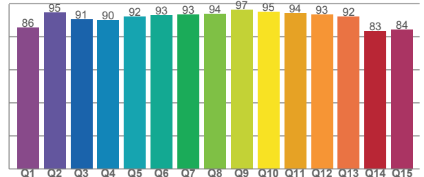
CQS: 90.5
