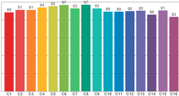
TM30: 91.1
